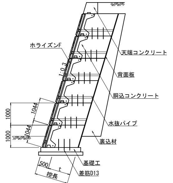
標準断面図
