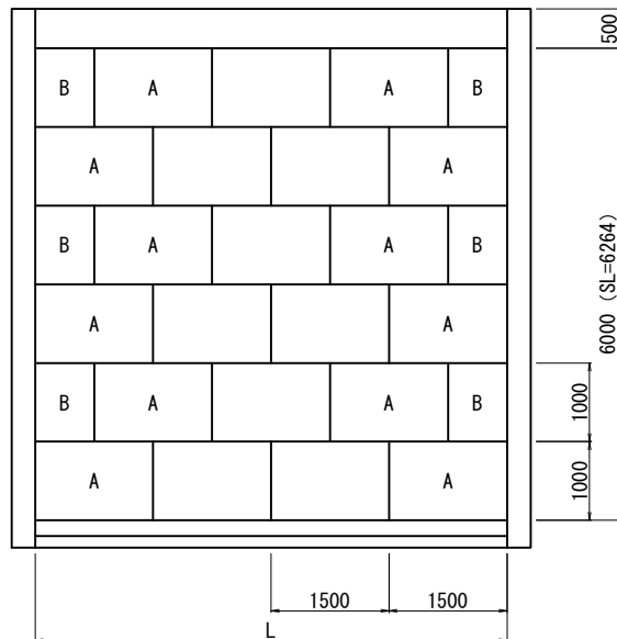
標準展開図
